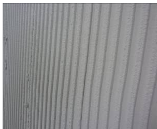
Рисунок 4.8. - Шаг 2. Нанесение при помощи зубчатой терки (величина зуба от 8-10 мм)
