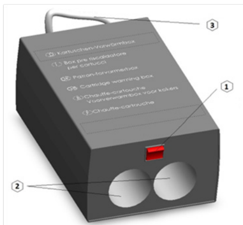
Slika 1: Pregrejač 2-Pipe kertridža TEROSON ET CR Heatingbox 2 CR
