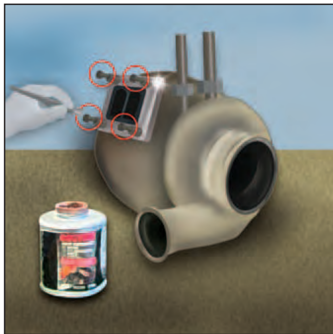
Środki smarne
