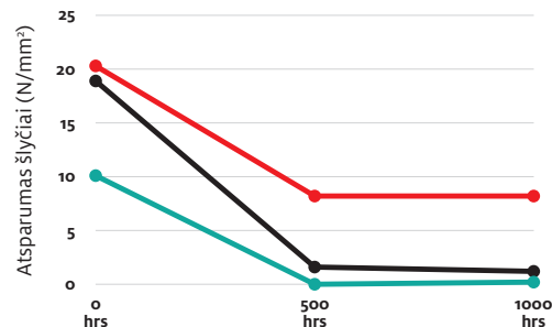
„LOCTITE 402“ Palyginimas su įprastiniais momentiniais kljais: atliekant terminį sendinimą 135 °C temperatūroje ir atsparumo šlyčiai bandymą ant nerūdijančio plieno kambario temperatūroje
