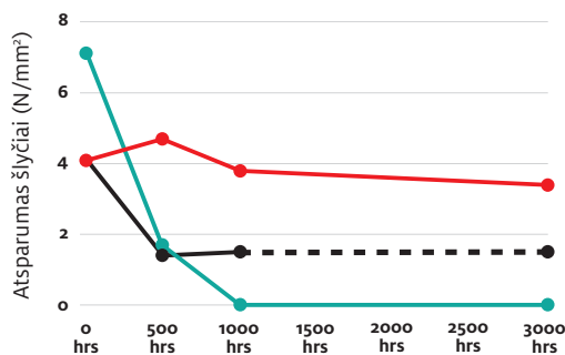
„LOCTITE 402“ Palyginimas su įprastiniais momentiniais kljais: atliekant terminį sendinimą 135 °C temperatūroje ir atsparumo šlyčiai bandymą ant nerūdijančio plieno 135 °C temperatūroje
