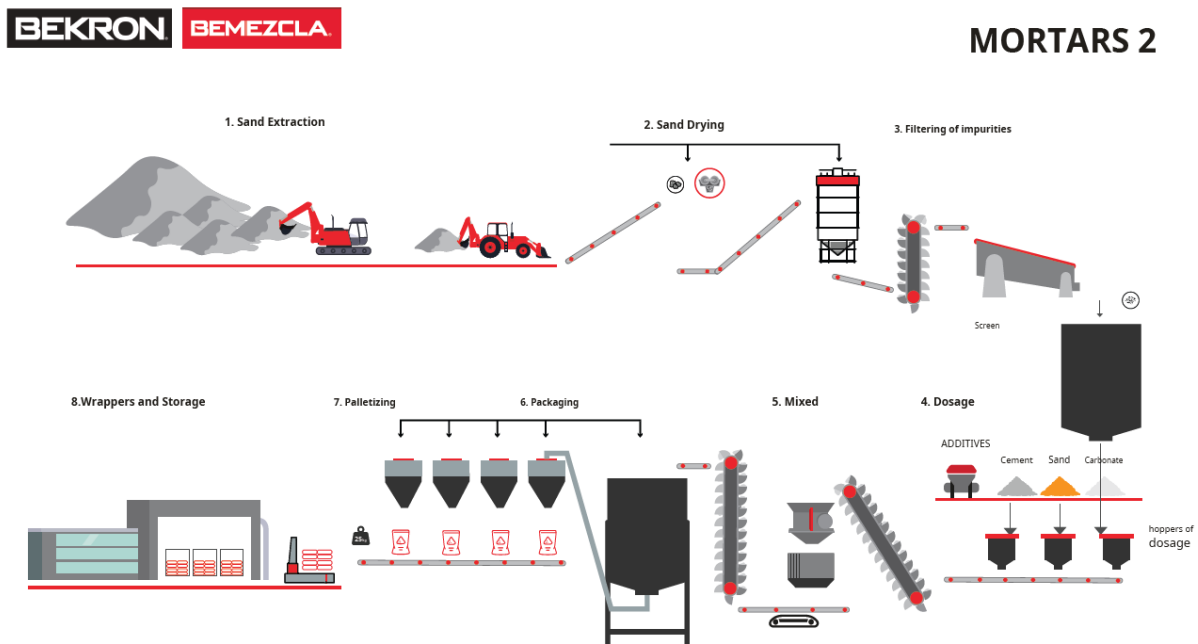
Figure 2. Flow diagram of the manufacturing process of Stucco products: Bemezcla CEM, Bemezcla FFL y Bemezcla FFL-i (Aislantes Nacionales SPA, 2023).
