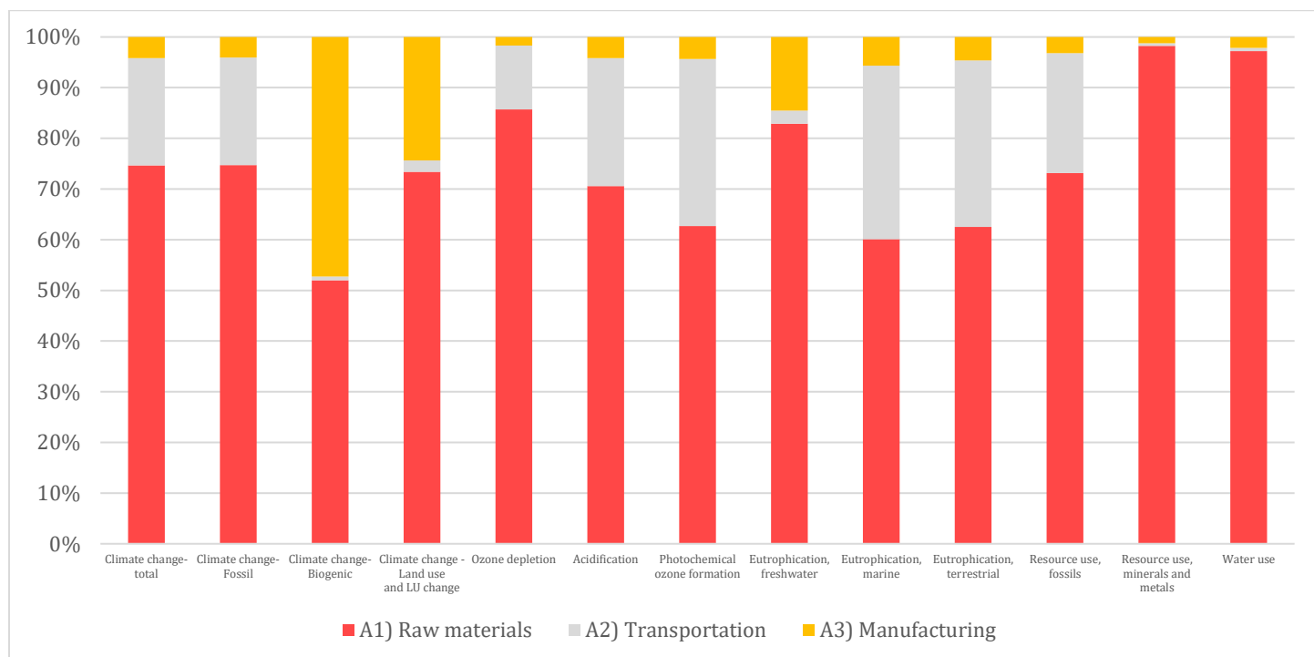
Figure 3. A1-A3 Basic impact categories results of Bemezcla Nivelación GL Fino
