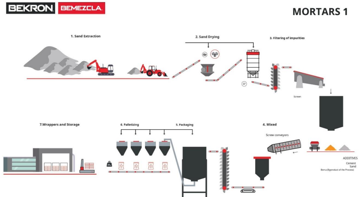
Figure 1. Flow diagram of the manufacturing process of of Bemezcla Leveling products: Bemezcla Nivelación GL and Bemezcla Nivelación GL fino (Aislantes Nacionales SPA, 2023).
