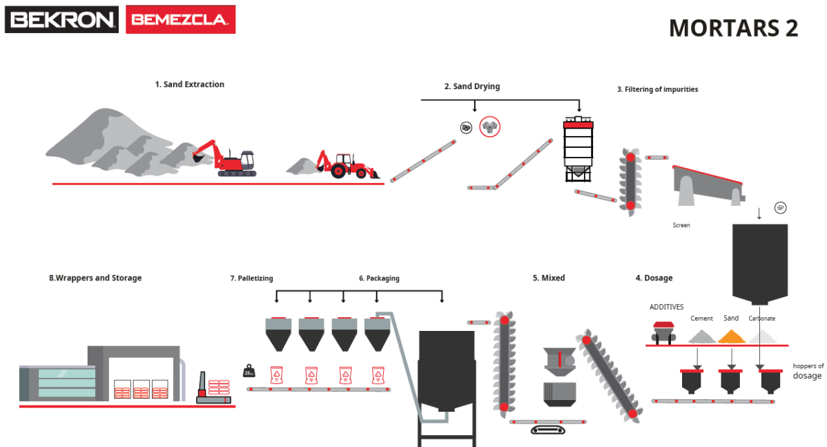
Figure 2. Flow diagram of the manufacturing process of Stucco products: Bemezcla Nivelación y Retape Plus, Bemezcla Nivelación y Retape and Bemezcla Autonivelante XL (Aislantes Nacionales SPA, 2023).
