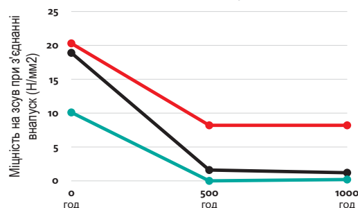
LOCTITE 402 ПОРІВНЯНО З ТИПОВИМИ МИТТЄВИМИ КЛЕЯМИ: ТЕРМІЧНА ВИТРИМКА ПРИ 135°C І ВИПРОБУВАННЯ МІЦНОСТІ НА ЗСУВ ПРИ З'ЄДНАННІ ВНАПУСК НА НЕРЖАВІЮЧІЙ СТАЛІ ПРИ КІМНАТНІЙ ТЕМПЕРАТУРІ
