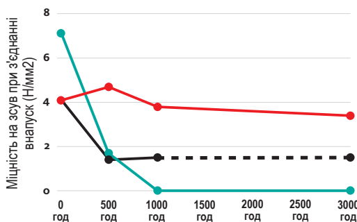
LOCTITE 402 ПОРІВНЯНО З ТИПОВИМИ МИТТЄВИМИ КЛЕЯМИ: ТЕРМІЧНА ВИТРИМКА ПРИ 135°C І ВИПРОБУВАННЯ МІЦНОСТІ НА ЗСУВ ПРИ З'ЄДНАННІ ВНАПУСК НА НЕРЖАВІЮЧІЙ СТАЛІ ПРИ 135°C
