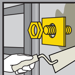
Akaszók, konzolok felszerelése a fürdőszobai felszerelésekhez
