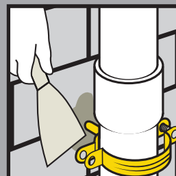
Vízvezeték tartóbilincsek rögzítése
