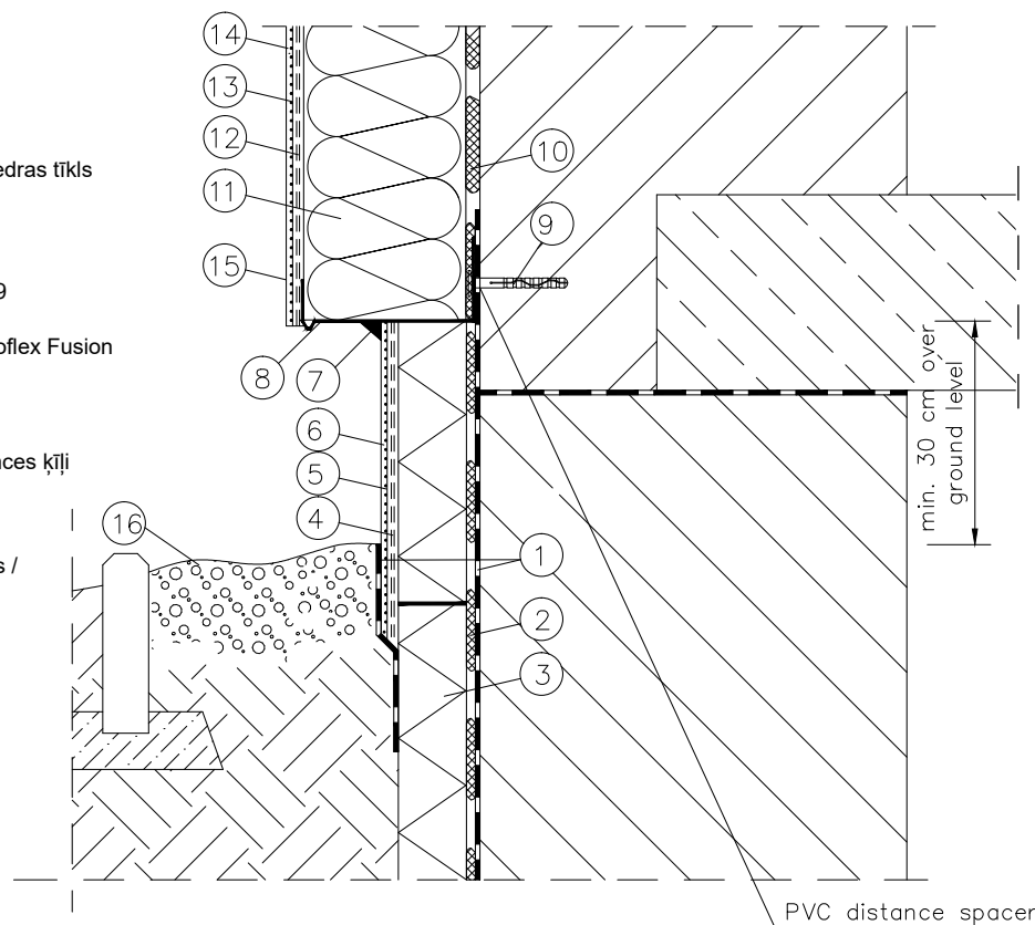
3. zīmējums. Ceresit Ceretherm ETICS sistēmas cokola un pandusa griezumums.
