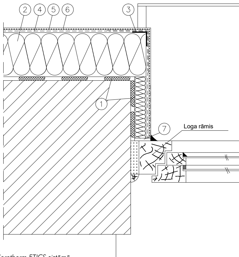
4. zīmējums. Loga zonas risinājums Ceretherm ETICS sistēmā
