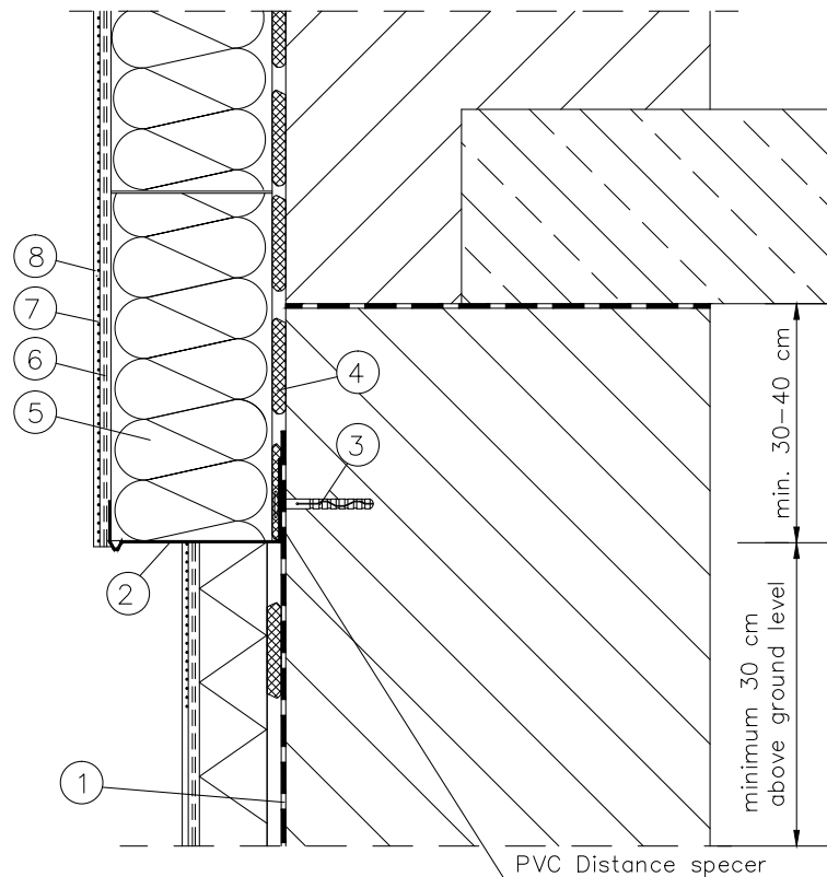
2. zīmējums. Ceresit Ceretherm ETICS minerālvates savienojums ar cokolu.
