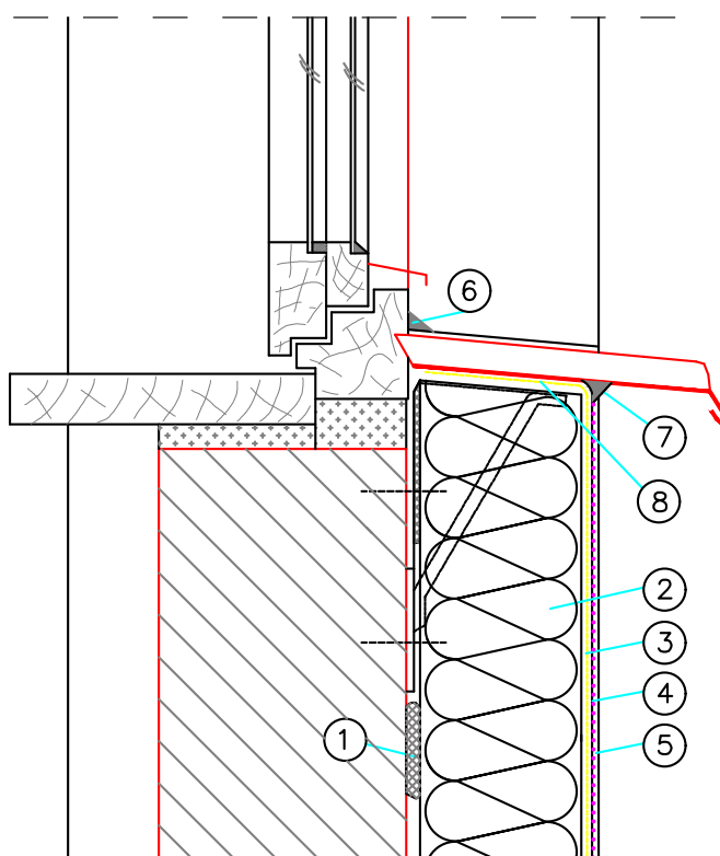
6. zīmējums. Palodzes un loga skārda risinājums Ceretherm ETICS sistēmā
